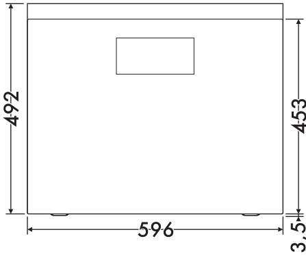
(вид спереди)
